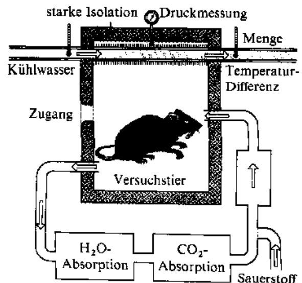
Das Prinzip der direkten Kalorimetrie
